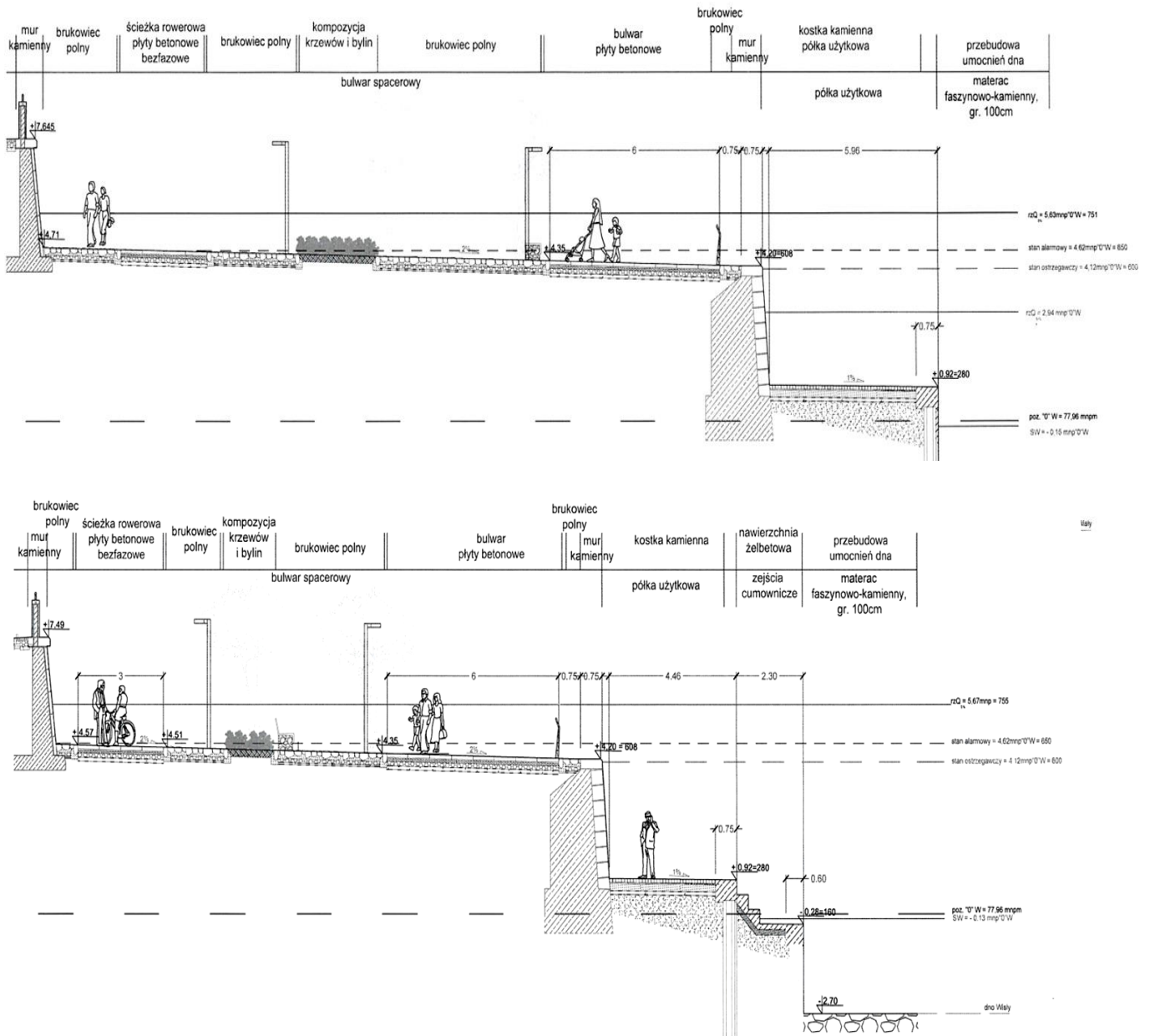
Szkic nr 2 - układ pionowy nabrzeża bulwaru Jana Karskiego.
