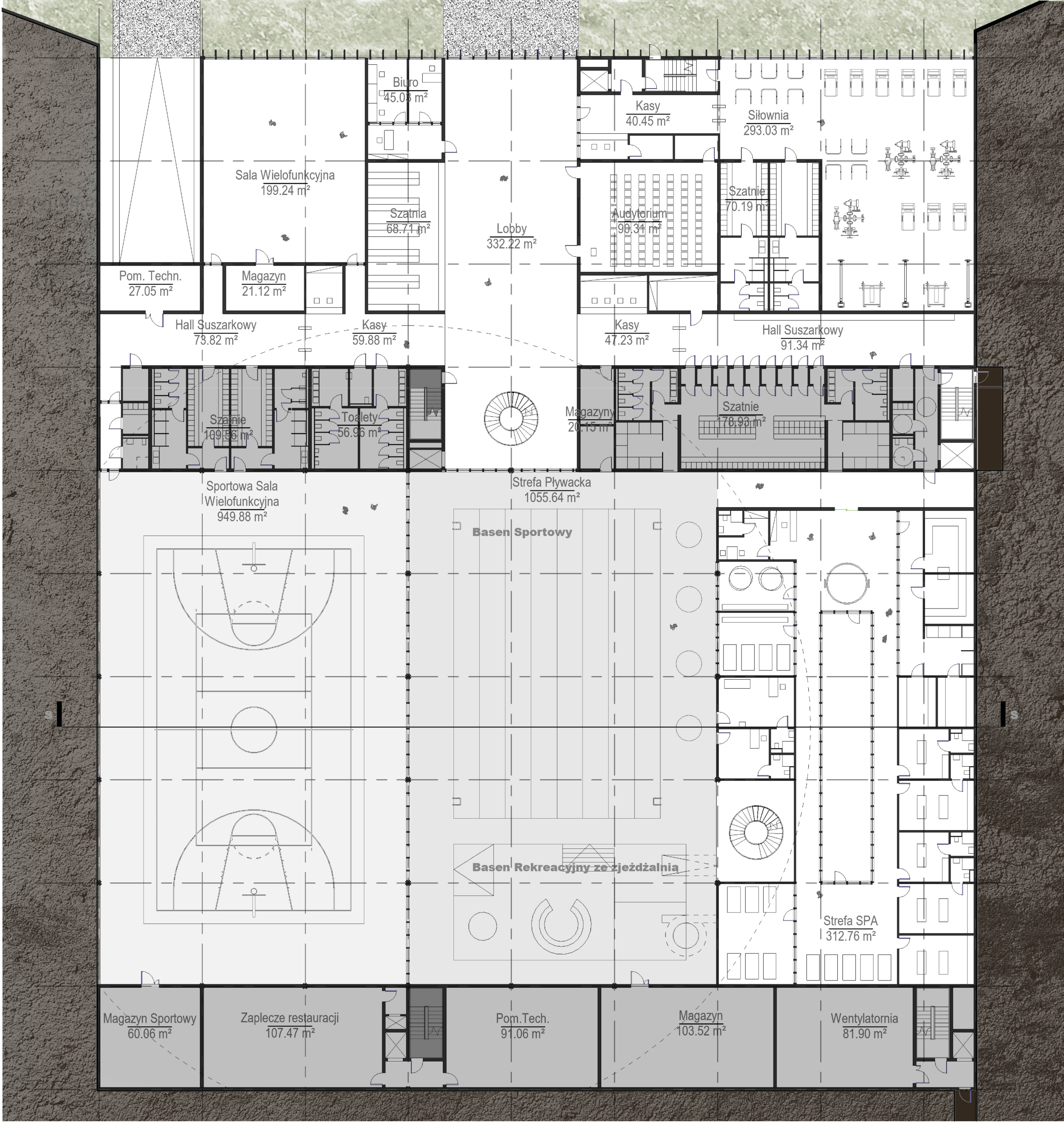
rzut parteru zespołu sportowego 1:500
