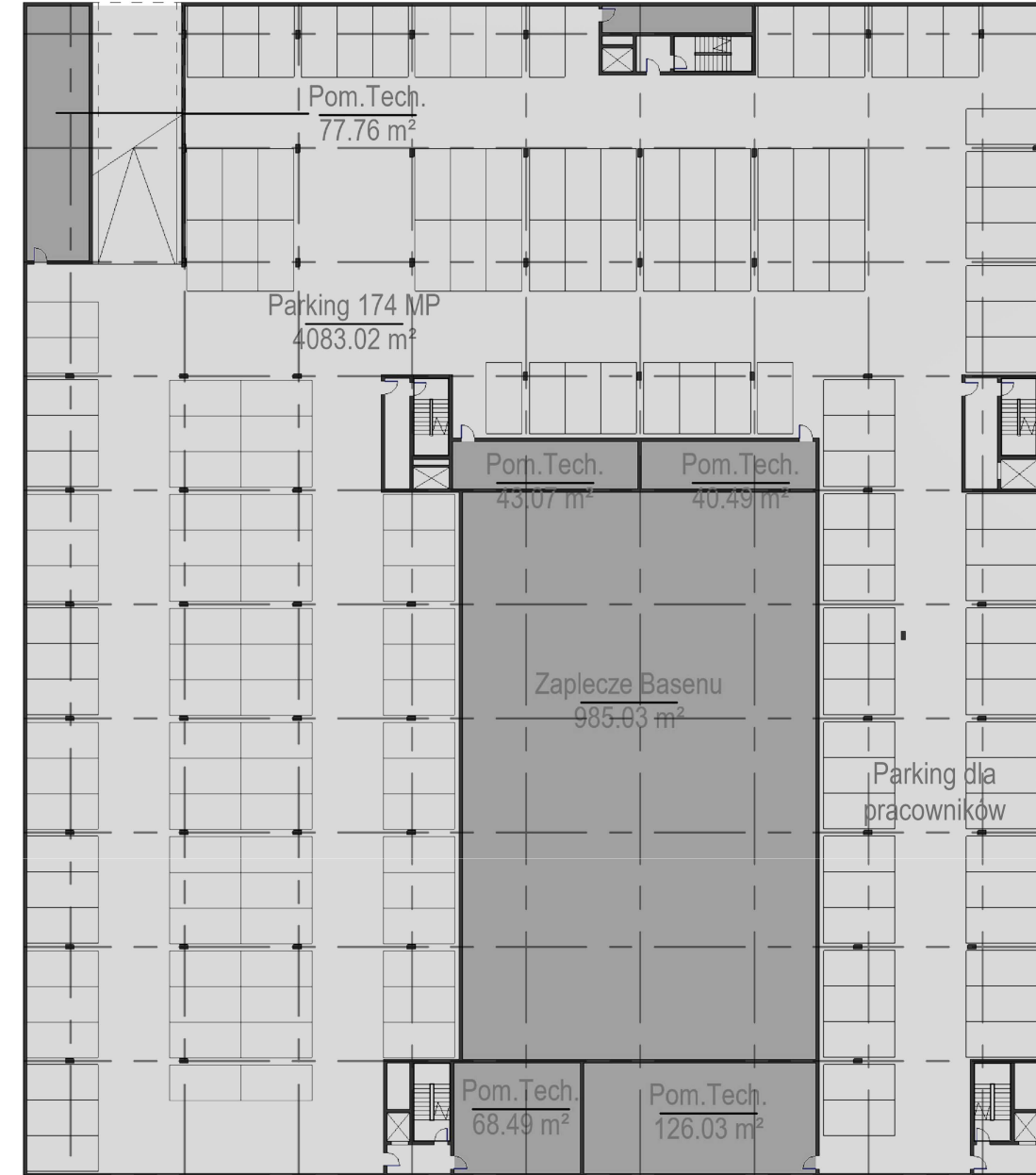
rzut parkingu zespołu sportowego 1:500
