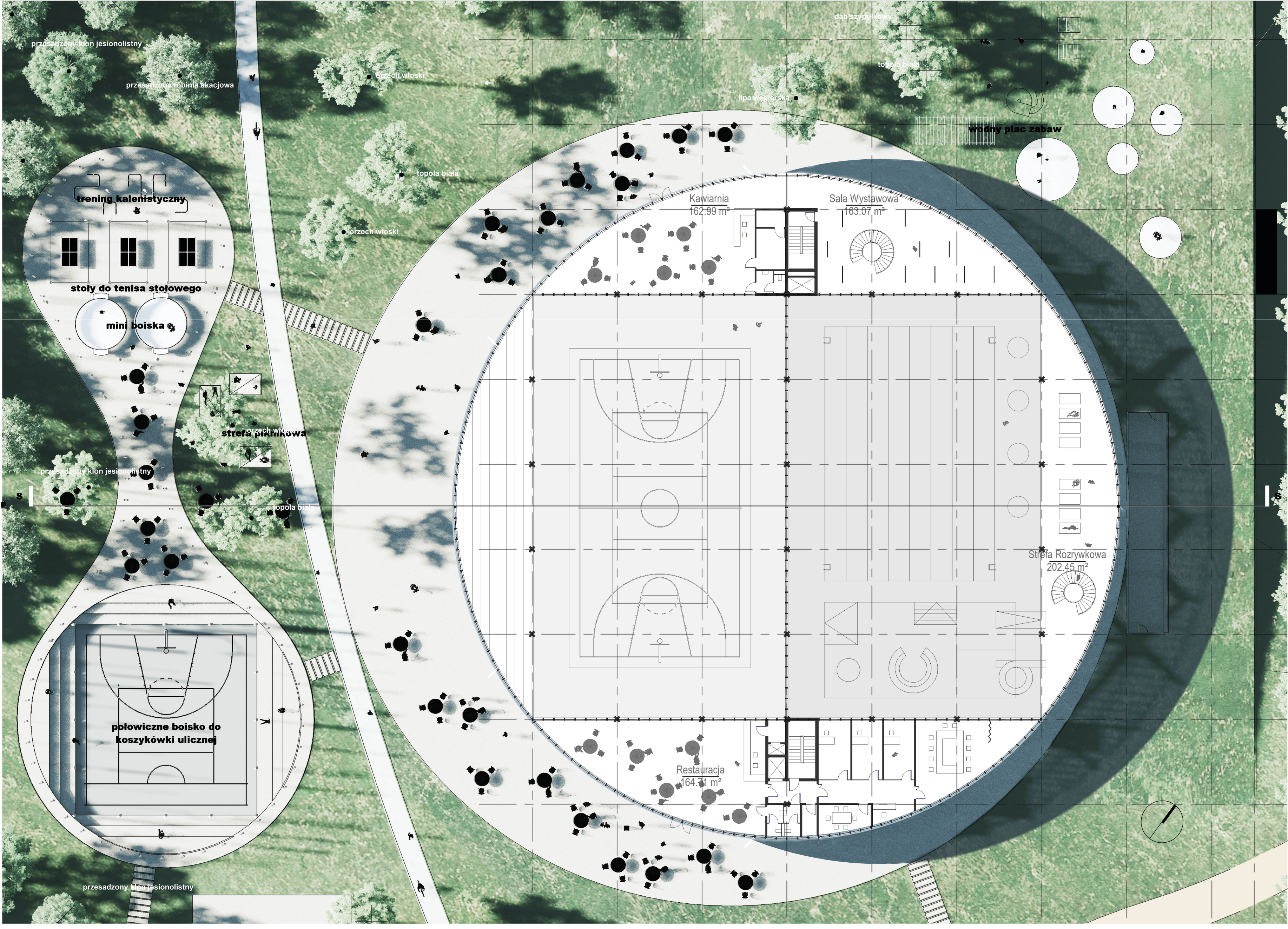
rzut pawilonu piknikowego oraz I. piętra zespołu sportowego 1:250
