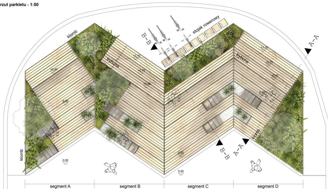
rzut parkletu - 1:50
